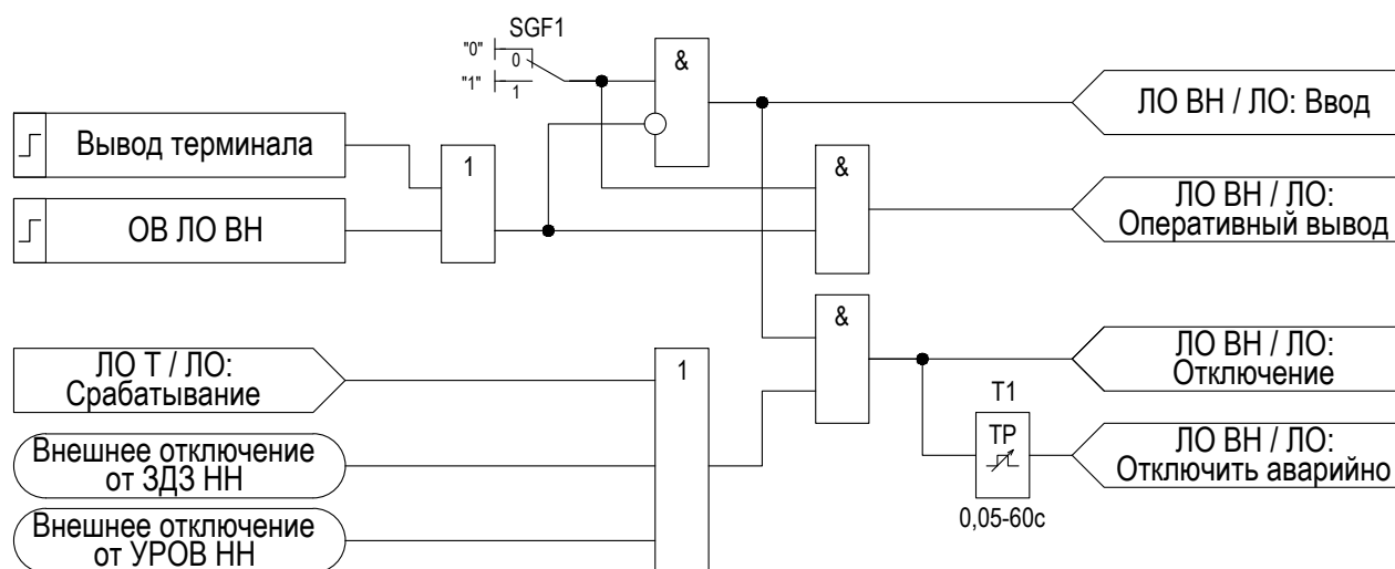
Рисунок 2.22 – Функциональная схема ЛО ВН
