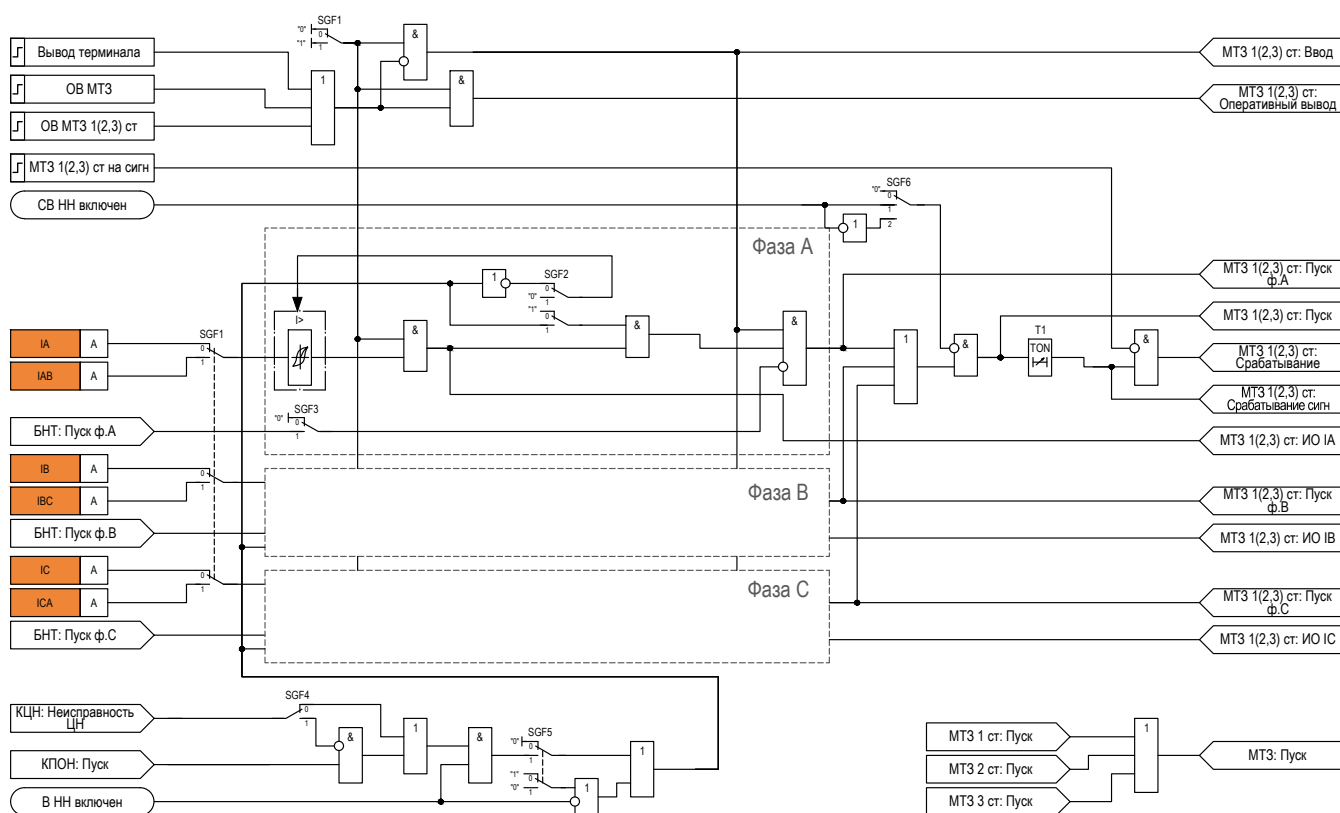
Рисунок 2.1 – Функциональная схема логики ступеней МТЗ
