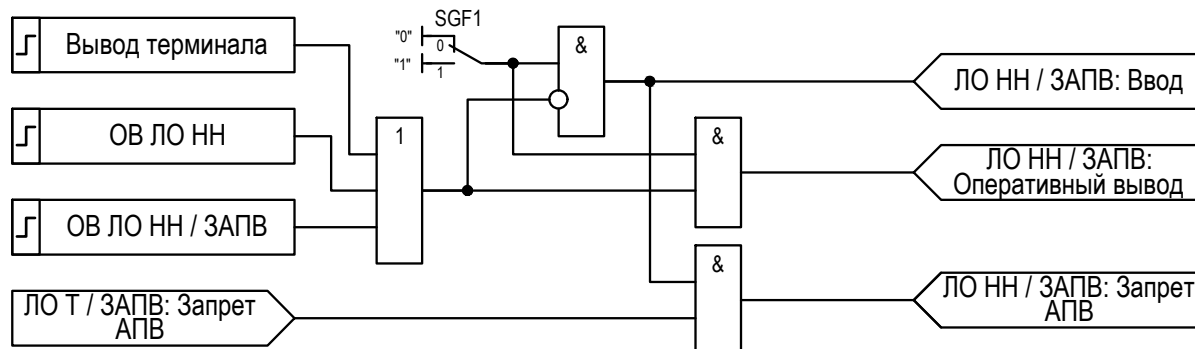
Рисунок 2.24 – Функциональная схема логики запрета АПВ
